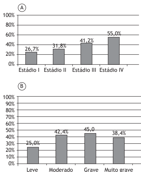
Figura 2. Prevalência de sarcopenia, diagnosticada por absorciometria de dupla energia por raios X, entre os pacientes com DPOC ( N = 91 ), segundo a gravidade da DPOC (estádios GOLD, em A) e o grau de obstrução ( VEF_1 , em B). Não houve correlação significativa da sarcopenia com os estádios GOLD ( p = 0,305 ) ou o VEF_1 ( p = 0,599 ). Grau de obstrução ( VEF_1 ): Leve ( \geq 80\% ); Moderado (50-79%); Grave (30-49%); e Muito grave ( < 30\% ).
